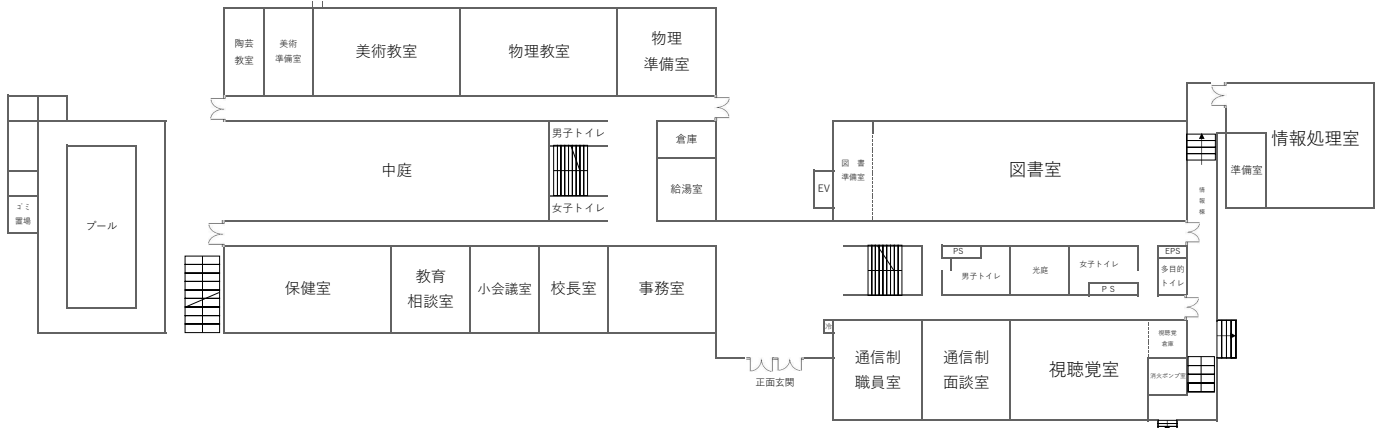
(1階平面図)
