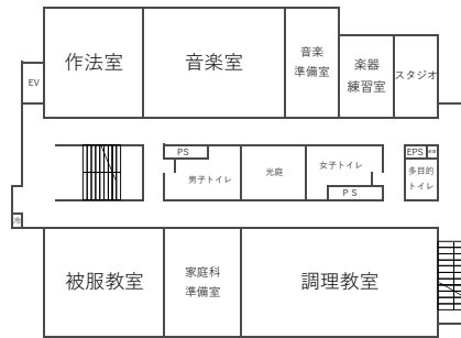
(5階平面図)
