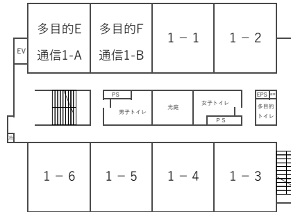
(4階平面図)
