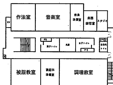
(5階平面図)
